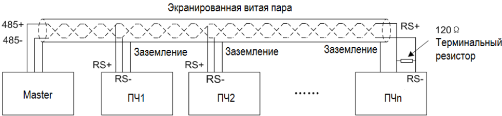
Схема сети с одним Master/несколькими Slave:
