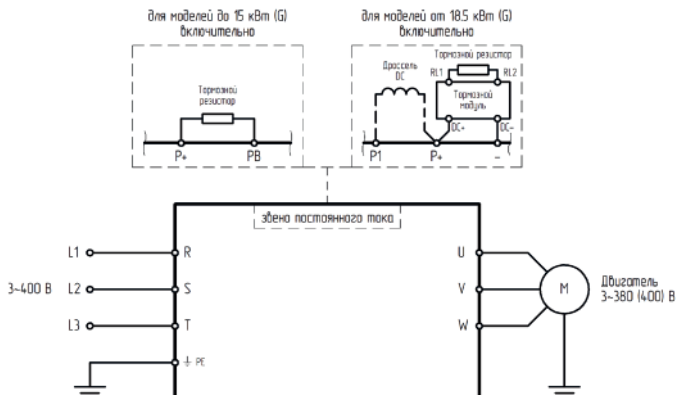
Рис. 2 – Подключение силовых клемм
