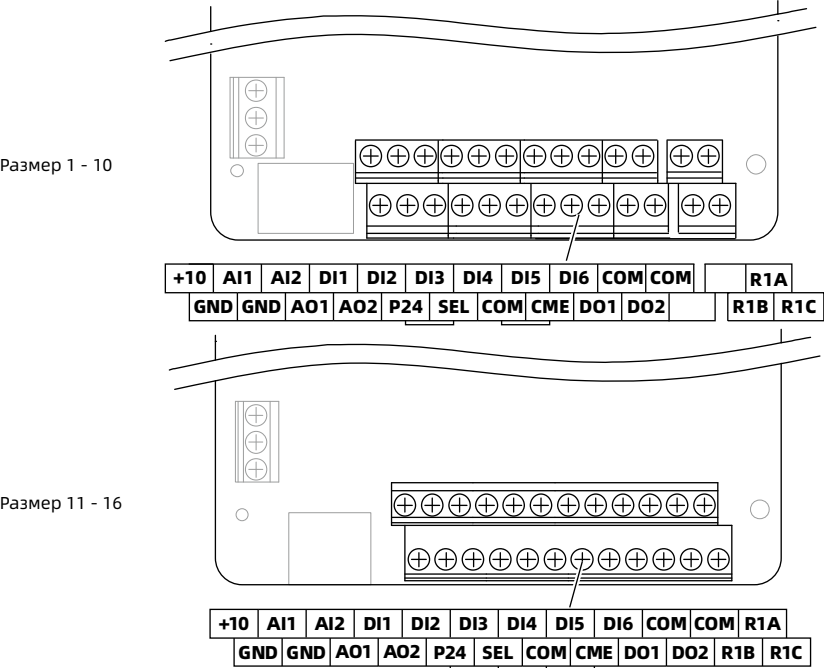
Рисунок 4-1 Клеммы управления
