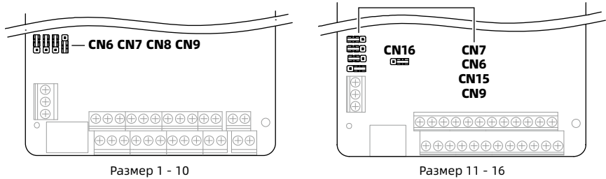
Рисунок 4-2 Расположение перемычек
