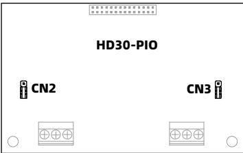
Рисунок 8-6 Расположение перемычек
