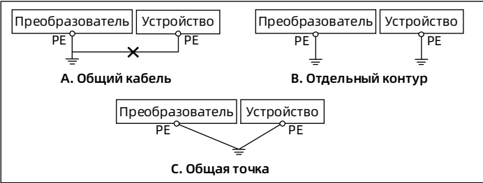
Рисунок 4-14 Варианты заземления
