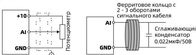
Рисунок 4-7 Схема подключения AI1
