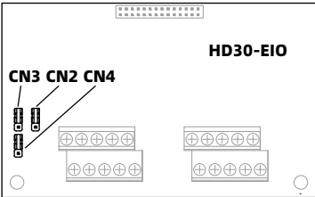
Рисунок 8-2 Расположение перемиычек Таблица 8-2 Описание перемиычек
