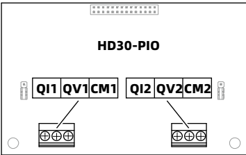
Рисунок 8-5 Расположение клемм HD30-PIO
