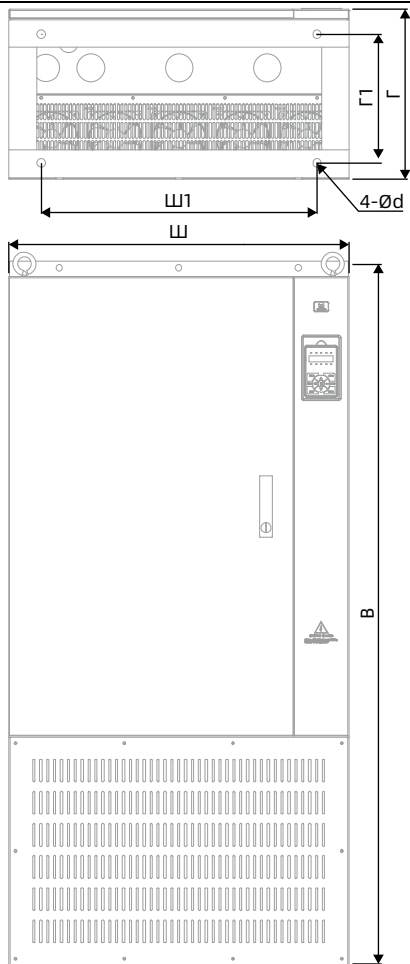
Рисунок 3-1 Преобразователь HD30 на напольной стойке (индекс -С)
