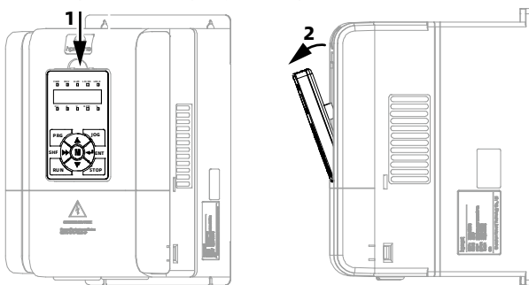
Рисунок 3-3 Снятие пульта
