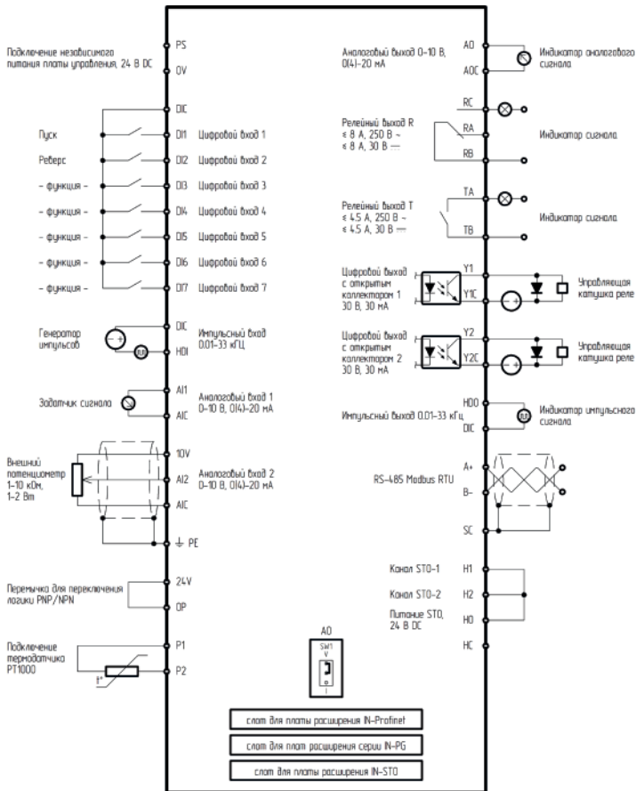
Рисунок 3 – Подключение управляющих клемм для преобразователя частоты серии INPRIME (плата IN-I/O-A)
