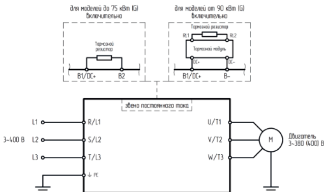
Рисунок 2 – Подключение силовых клемм для преобразователя частоты серии INPRIME
