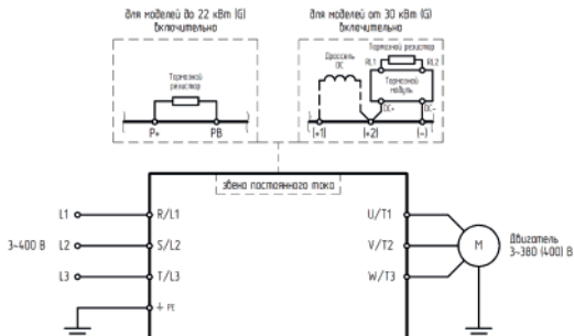
Рисунок 2г – Подключение силовых клемм
