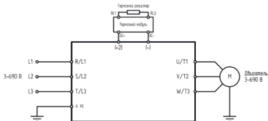
Рисунок 2д – Подключение силовых клемм
