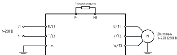
Рисунок 2б – Подключение силовых клемм
