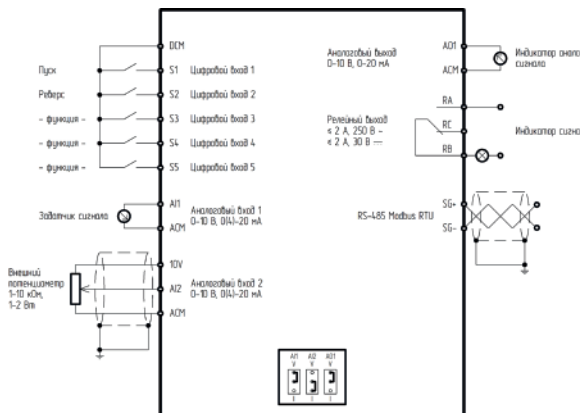
Рисунок 3 – Подключение управляющих клемм для преобразователя частоты серии LCI(S)
