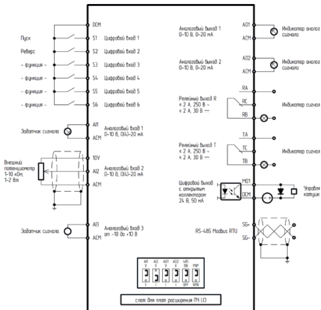
Рисунок 4 – Подключение управляющих клемм для преобразователя частоты серии LCI
