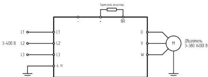
Рисунок 3 – Схема подключения трехфазных моделей NCI
