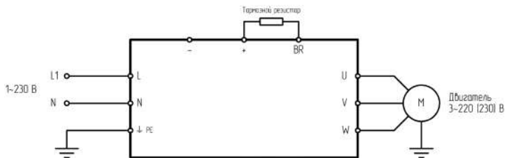
Рисунок 2 – Схема подключения однофазных моделей NCI
