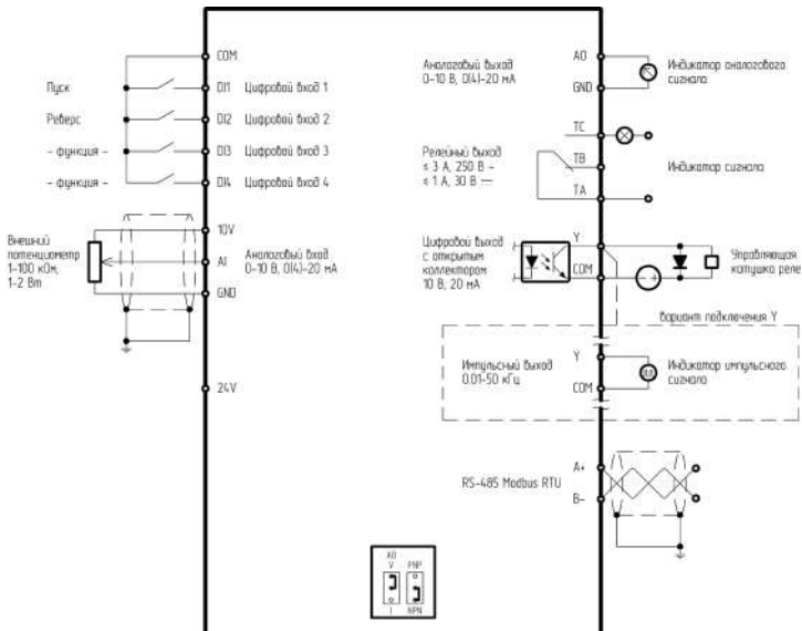
Рисунок 4 – Подключение управляющих клемм NCI
