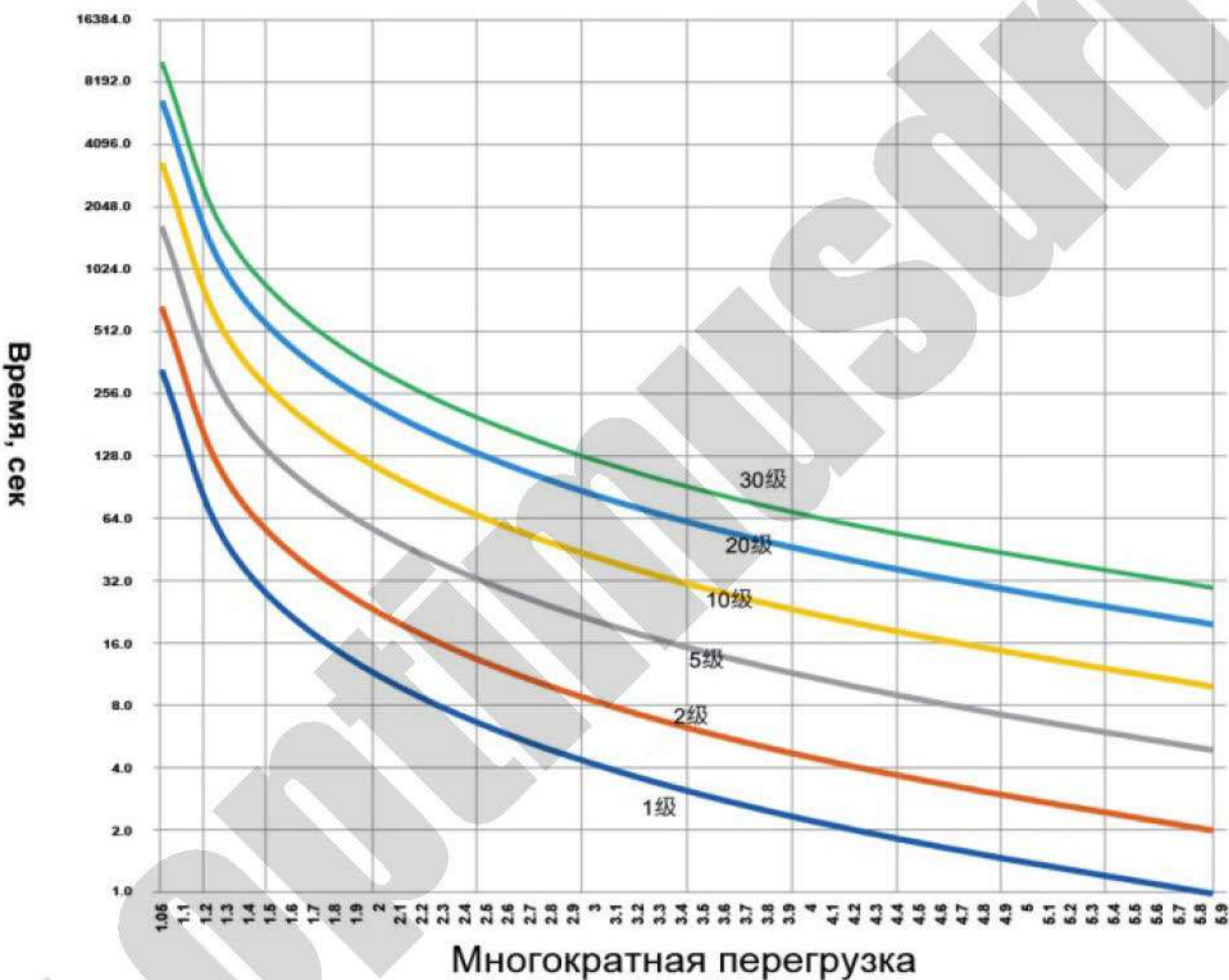
Характеристики защиты двигателя от перегрузки
