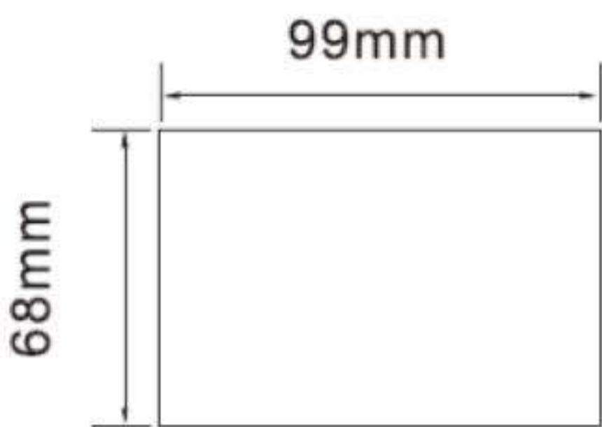
Рис. 1 Габаритные и монтажные размеры УПП (мм)
