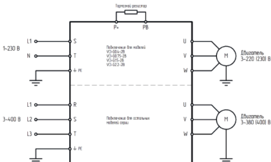
Рисунок 2 – Подключение силовых клемм
