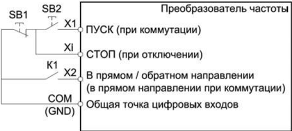
Рисунок 10.9-7. – Трёхпроводная схема управления 1
