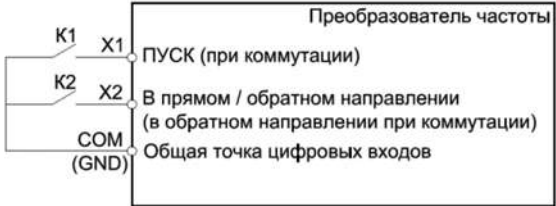
Рисунок 10.9-6. – Двухпроводная схема управления 2
