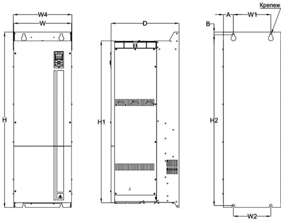
Рисунок 3.6-12 – Чертеж преобразователя частоты типоразмера B12
