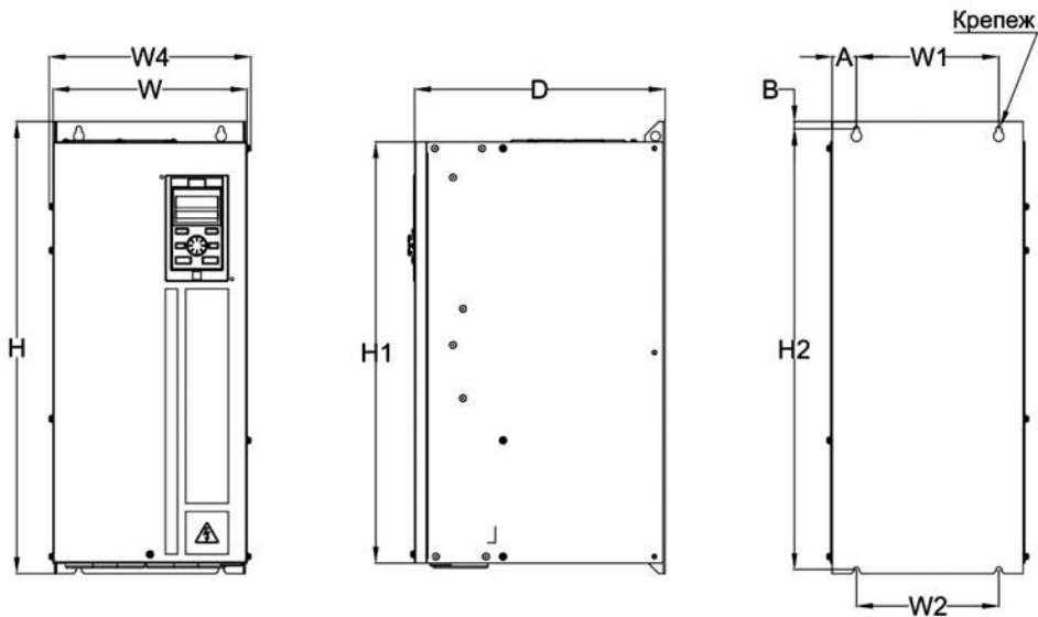
Рисунок 3.6-6 – Чертеж преобразователя частоты типоразмера B6
