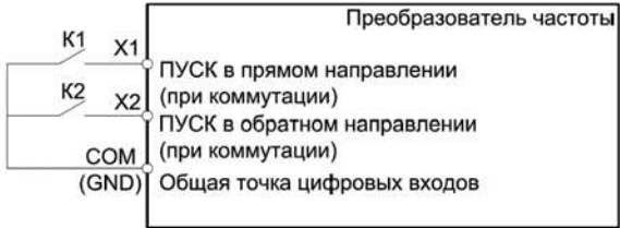
Рисунок 10.9-5. – Двухпроводная схема управления 1
