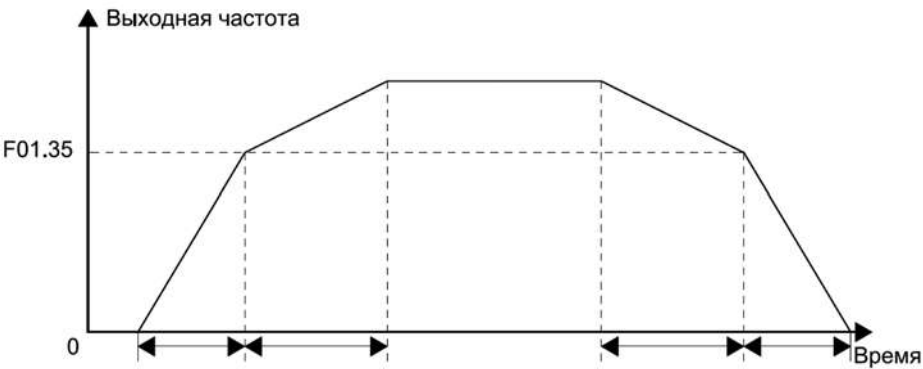
Рисунок 10.5-4 – Пример изменения выходной частоты при переключении между наборами параметров времени разгона и торможения при достижении заданной в параметре F01.35 частоты
