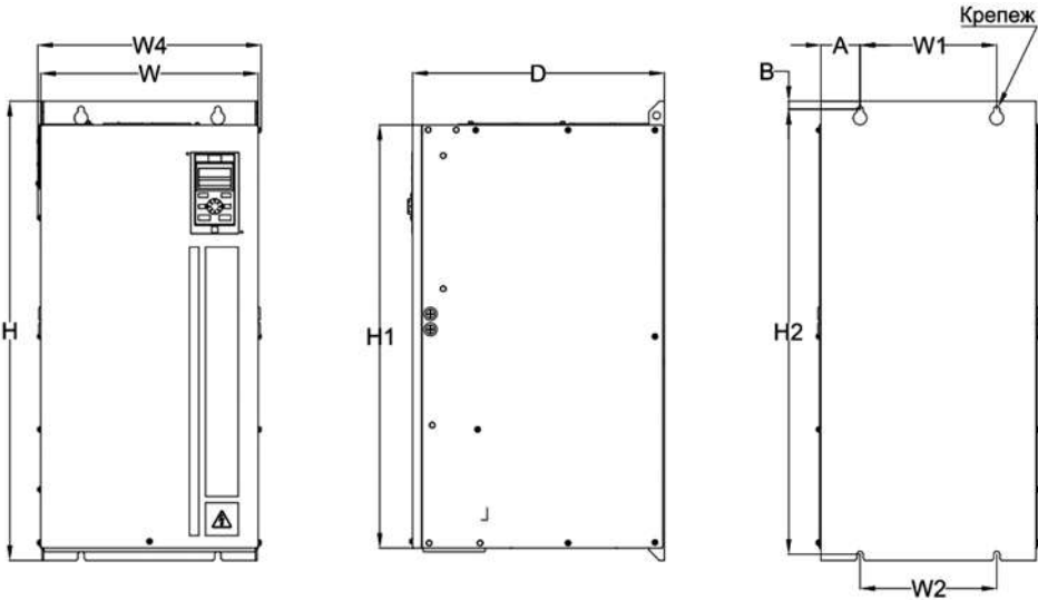
Рисунок 3.6-8 – Чертеж преобразователя частоты типоразмера В8
