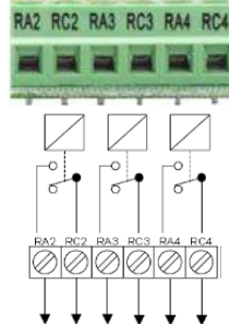
Три нормально-открытых контакта
