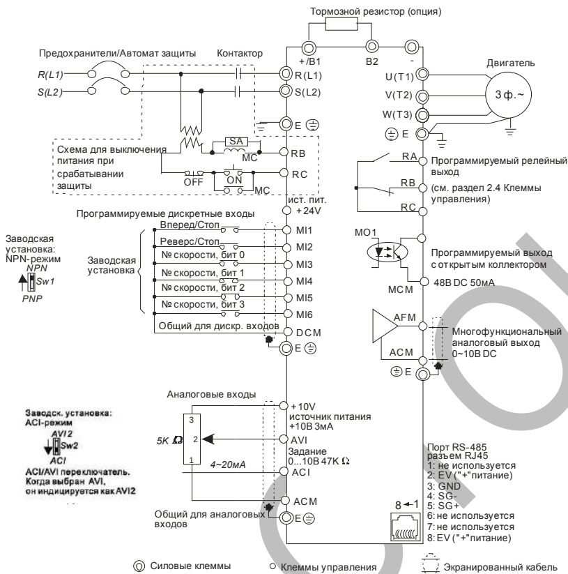
Рисунок 3. Схема для моделей
