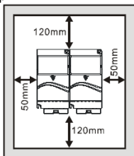
Метод установки В Типоразмер А
