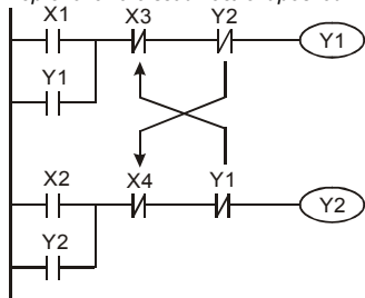
Пример 5: схема с взаимоблокировкой
