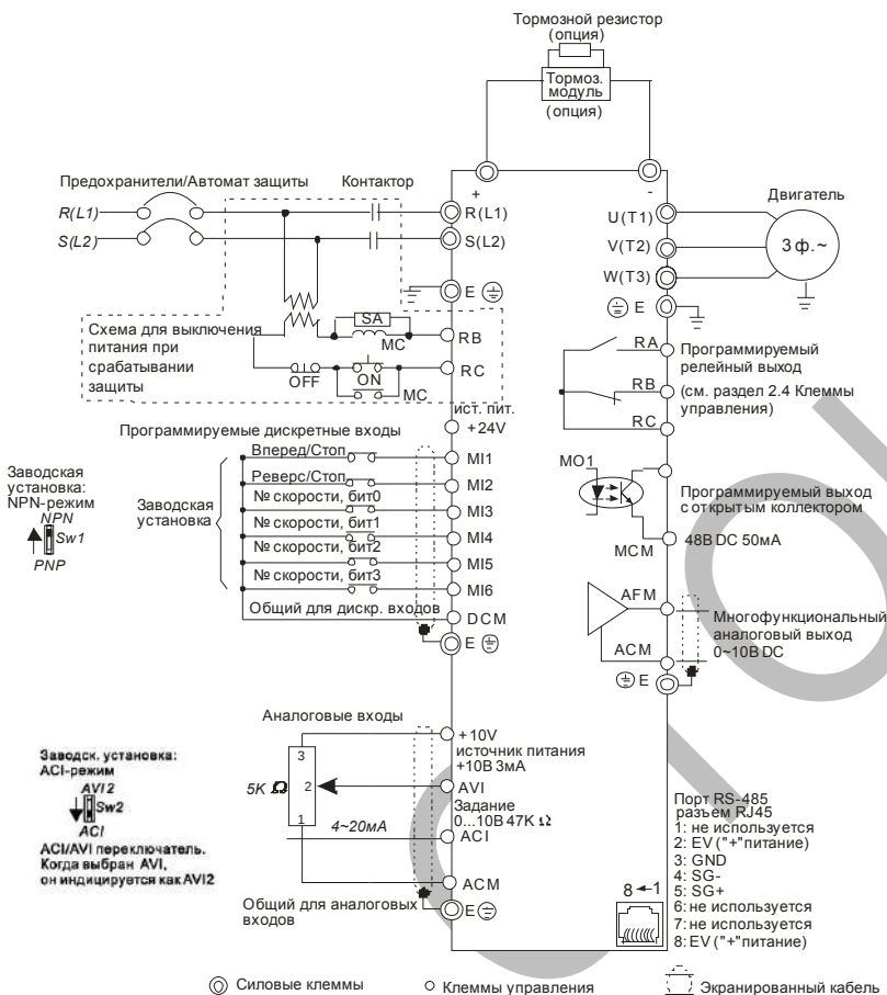
Рисунок 1. Схема для моделей
