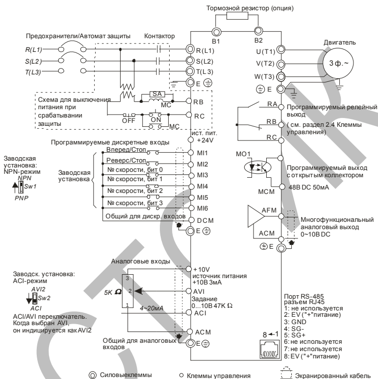
Рисунок 6. Схема для моделей VFD002E2 3T, VFD004E 23/43T, VFD007E23T/43T, VFD01523T/43T.
