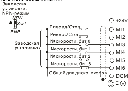
Рисунок 7. Выбор логики управления дискретными входами микропереключателем Sw1.
