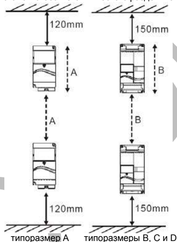
Установка без металлического разделителя
