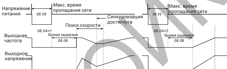
Рестарт после пропадания напряжения питания
